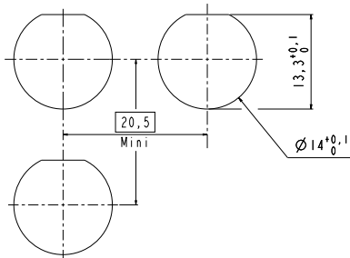
Jam nut receptacle 387TV*07***
