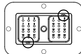
24 Pos Receptacle - Key B
