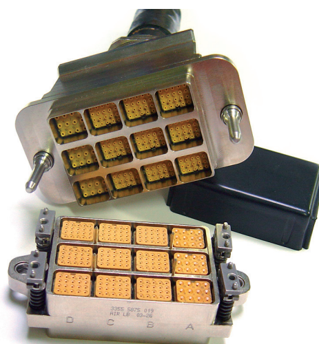
Connecteur rackable métallique 12 modules 12 modules metallic rackable connector
