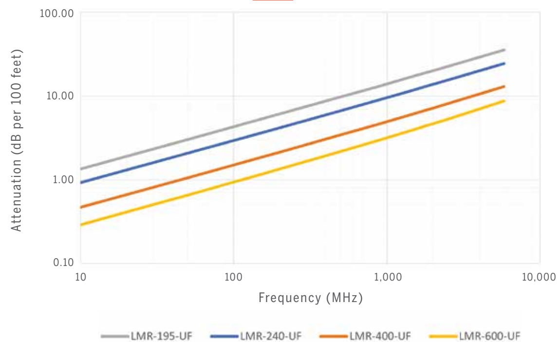
LMR UltraFlex
