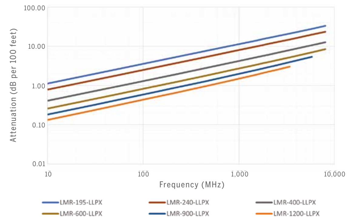
LMR LLPX
