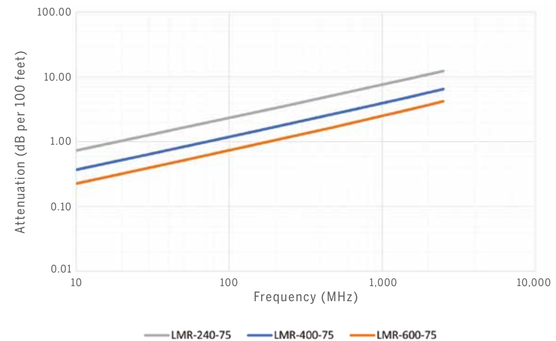
LMR 75 Ohm
