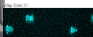
Ni K \alpha 1
