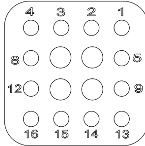
12+4 Way=12*#16+4*#12
