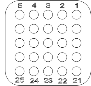
25 Way=25*#16
