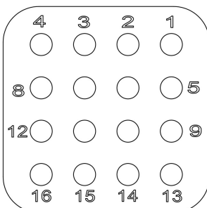
16 Way=16*#16
